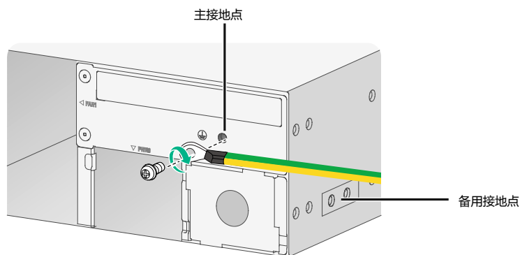
图2-4 连接接地线（以主接地点为例）
