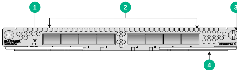
图A-9 NSQM1GP8A 接口模块正视图
