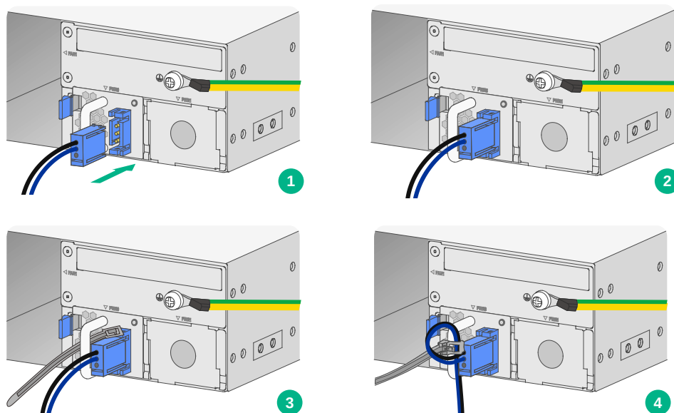
图2-16 连接直流电源线
