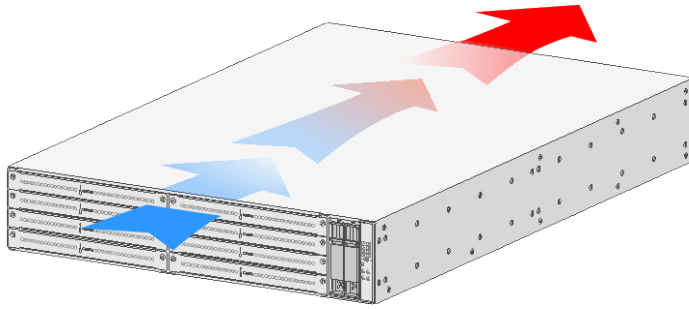
图1-2 设备安装 FAN-20B-2-A/FAN-80B-2-B 风扇模块
