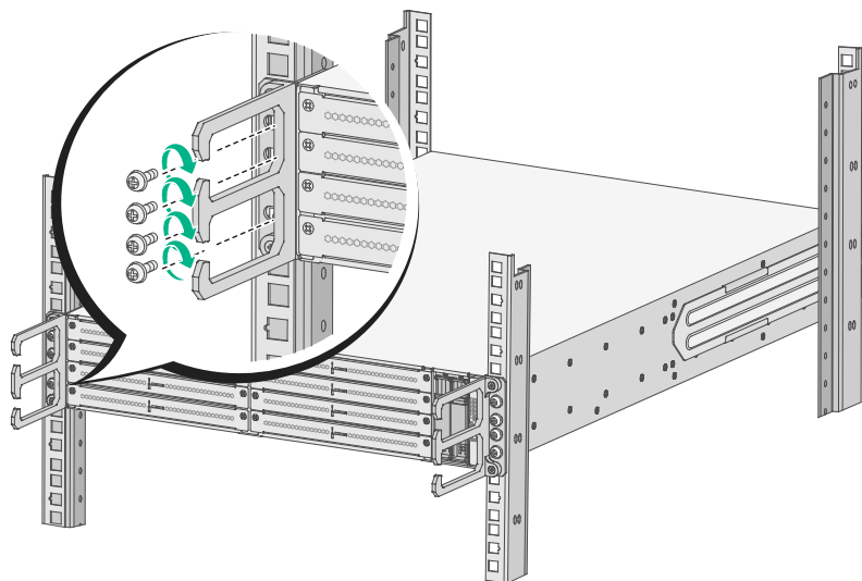
图2-3 安装设备到机柜
