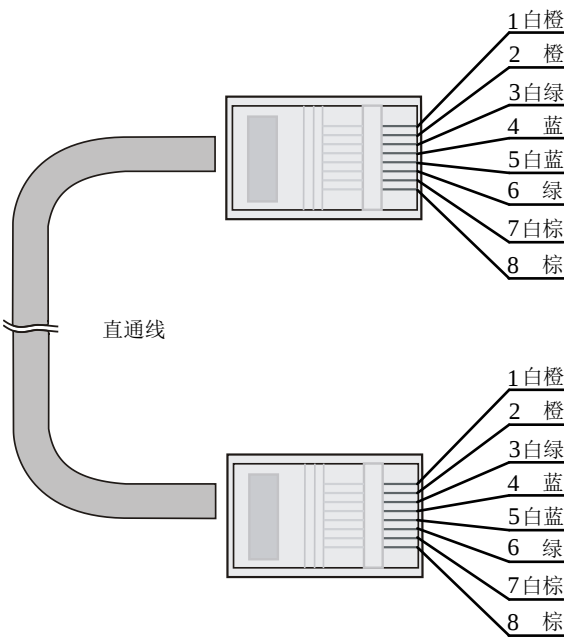
图C-4 直通线两端线序示意图
