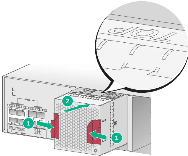
图2-7 风扇模块安装示意图
