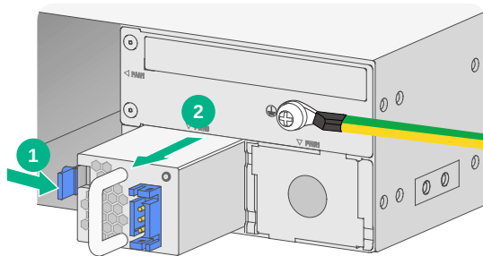
图4-3 拆卸电源模块（以直流电源模块为例）
