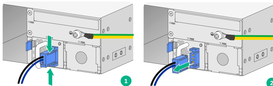
图4-2 拆卸电源线（以直流电源线为例）
