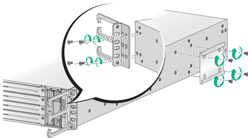
图2-2 安装前挂耳
