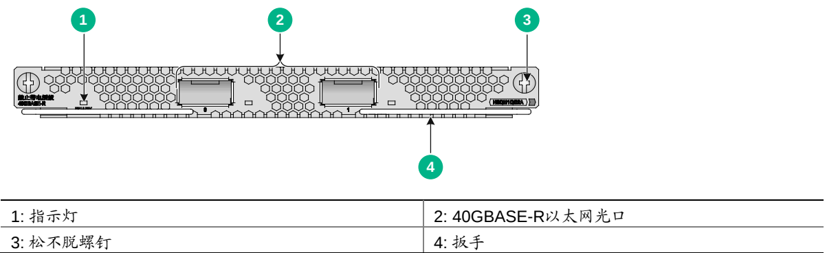
图A-6 NSQM1QG2A 接口模块正视图
