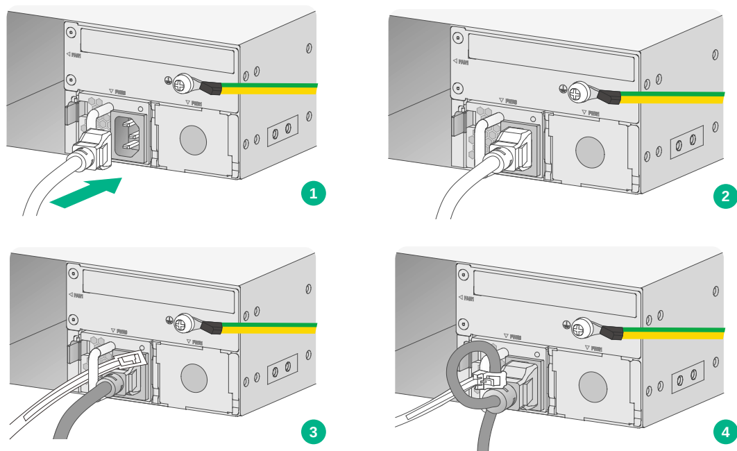
图2-15 连接交流电源线
