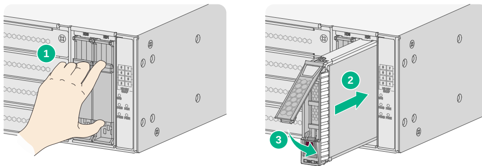
图2-9 安装硬盘
