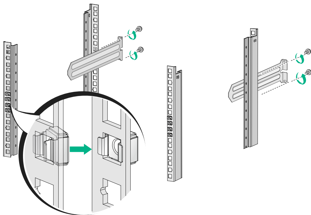
图2-1 安装浮动螺母及滑道
