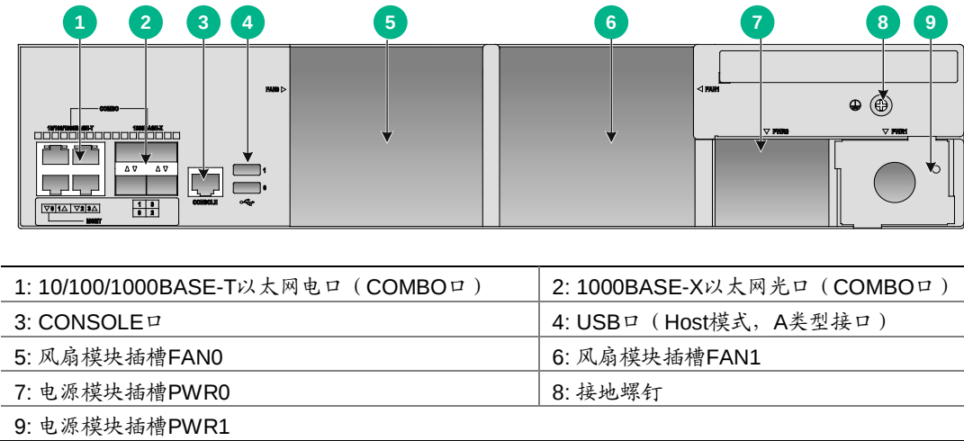
图A-4 设备后视图
