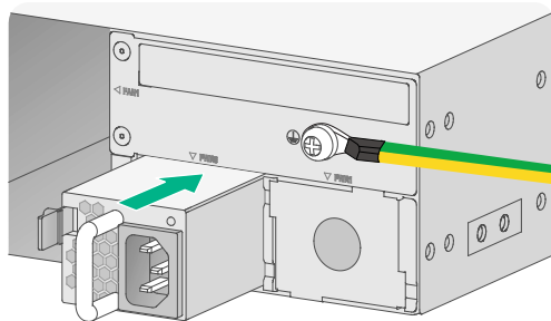
图2-5 安装电源模块（以交流电源模块为例）
