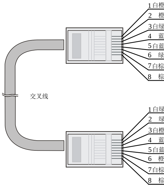
图C-5 交叉线两端线序示意图
