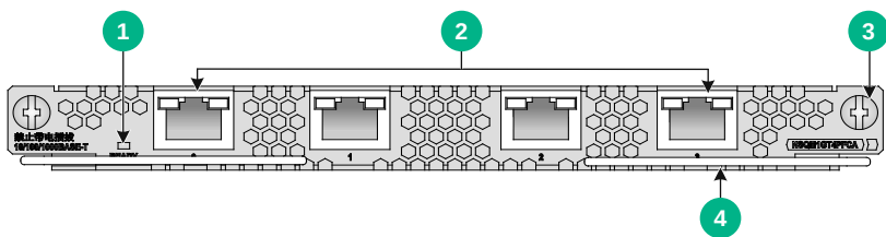
图A-10 NSQM1GT4PFCA 接口模块正视图
