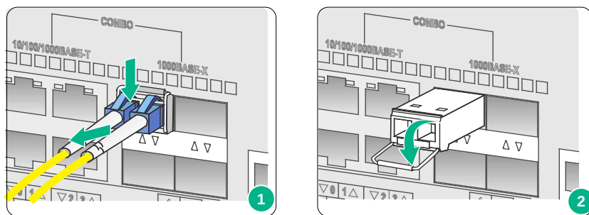
图4-6 拆卸光接口模块示意图
