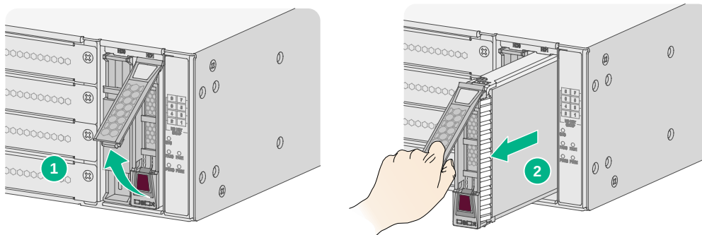
图2-10 拆卸硬盘
