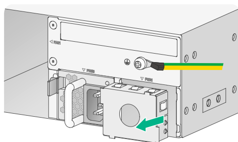
图2-6 拆卸电源槽位假面板
