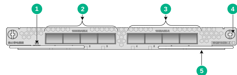
图A-7 NSQM1G4XS4-Z 接口模块正视图
