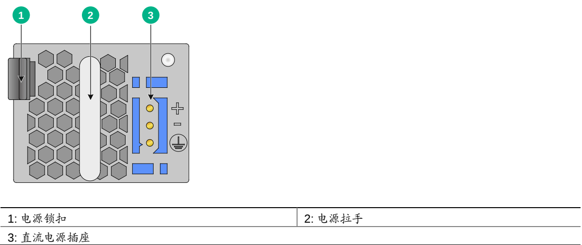
图A-12 直流电源模块正视图
