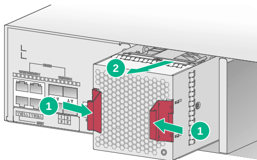
图4-1 风扇模块拆卸示意图
