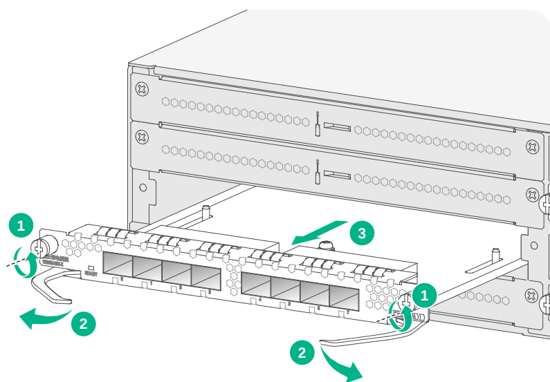
图4-4 拆卸接口模块
