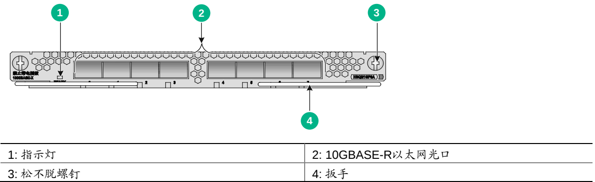
图A-5 NSQM1TG8A 接口模块正视图
