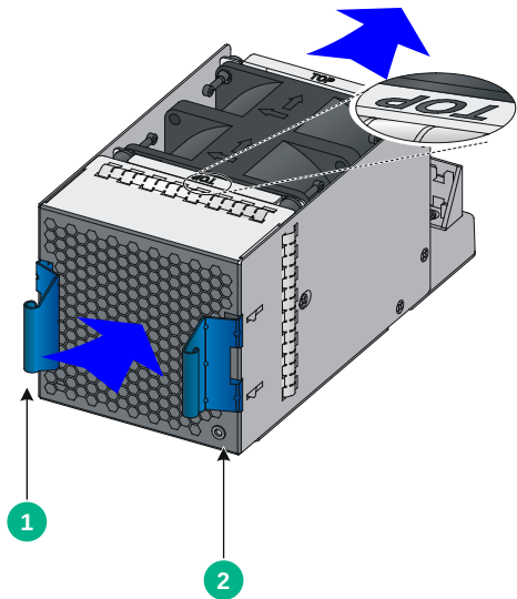
图A-13 FAN-20F-2-A/FAN-80F-2-B 外观图
