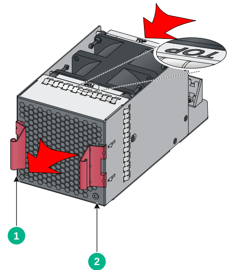
图A-14 FAN-20B-2-A/FAN-80B-2-B 外观图
