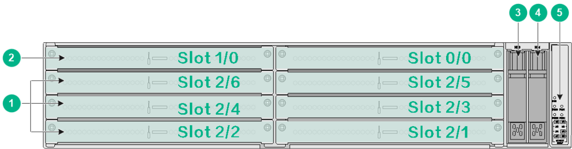
图A-3 设备前视图
