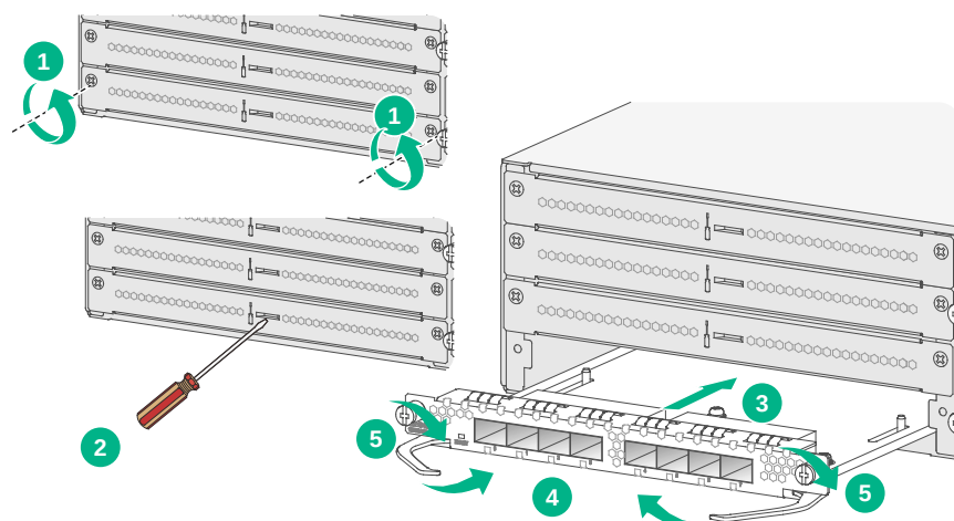
图2-8 安装接口模块
