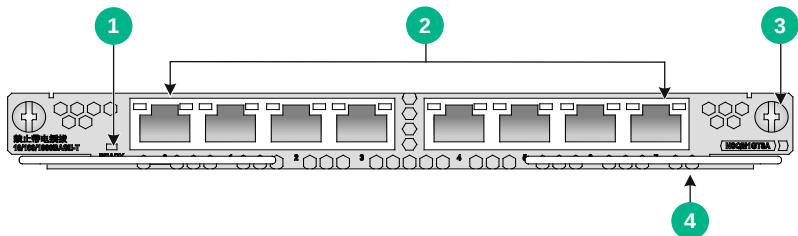
图A-8 NSQM1GT8A 接口模块正视图
